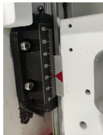
Belka dociskowa z 2 prowadnicami pryzmatycznymi
