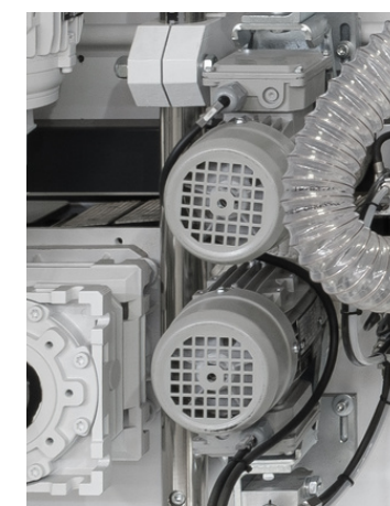
Stacja polerowania Opcjonalnie
